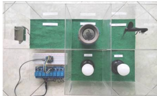
Gambar 2. Rangkaian Menggunakan Peralatan Elektronik
